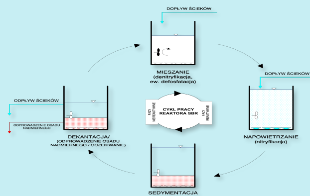
Fazy w cyklu oczyszczania reaktora SBR
